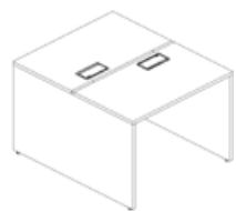
PLATAFORMA INICIAL DUPLA PAINEL PROF. 1400 mm
